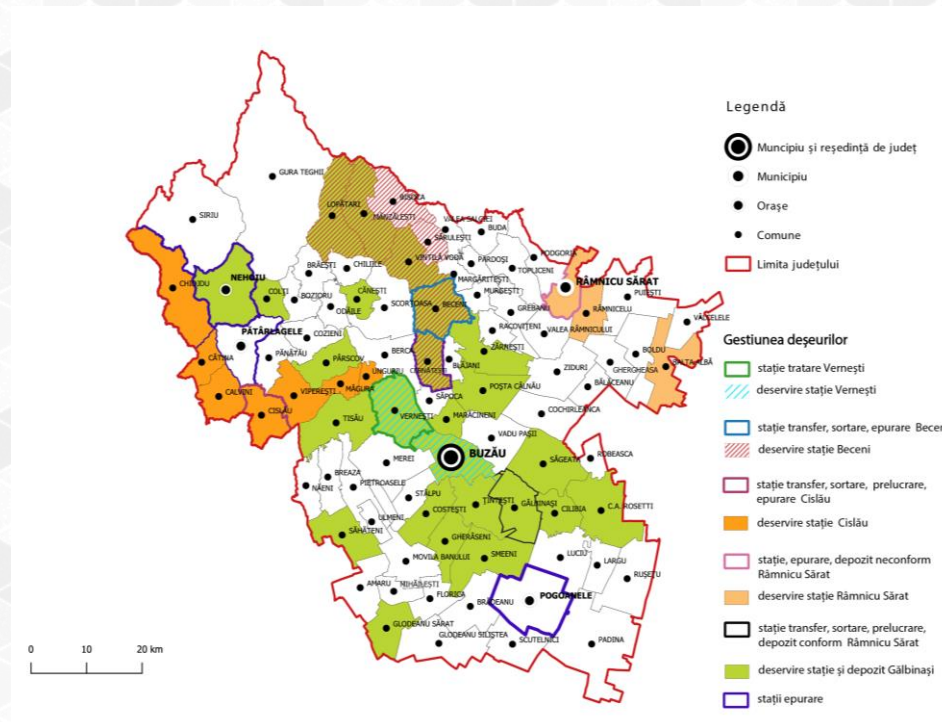
Figura nr. 31 – Harta infrastructurii de gestiune a deșeurilor de la nivelul județului Buzău
