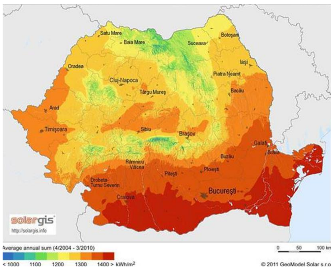
FIGURĂ 78 - IRADIAȚIA GLOBALĂ ORIZONTALĂ ÎN ROMÂNIA
