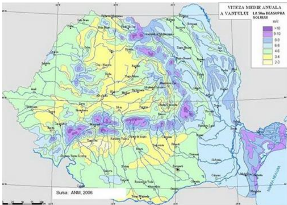
FIGURĂ 79 - VITEZA MEDIE ANUALĂ A VÂNTULUI LA 50 M DEASUPRA SOLULUI ÎN ROMÂNIA
